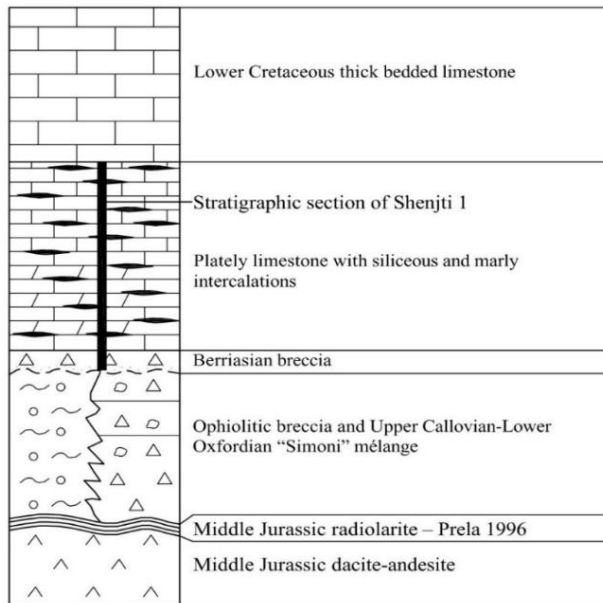
Fig. 3-1: Stratigraphic column of Nenshenjüt.
