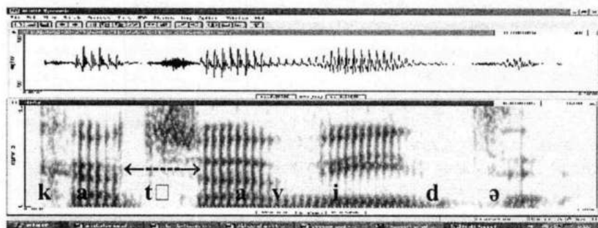
La forme de l'onde et le spectrogramme du mot kaçavidë .
